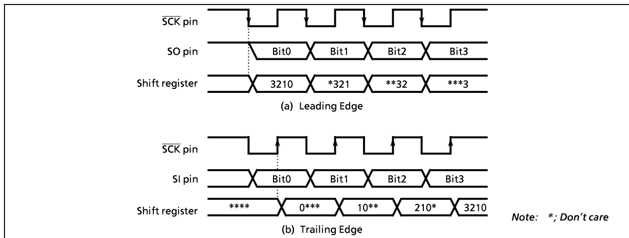
Figure 2-32. Shift Edge
